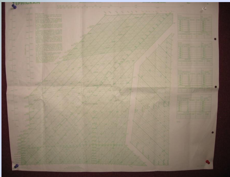
Mo2810A - Tephigram
